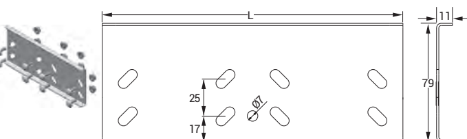
СОЕДИНИТЕЛЬНЫЙ ЭЛЕМЕНТ 075 СТЕ
