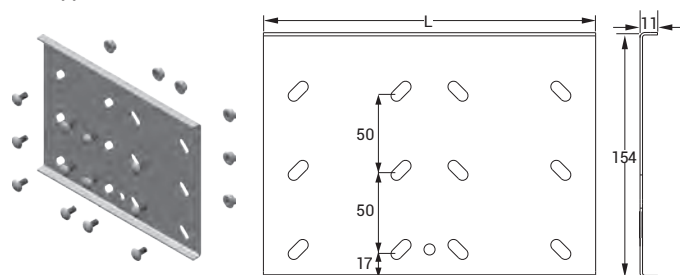
СОЕДИНИТЕЛЬНЫЙ ЭЛЕМЕНТ 150 СТЕ
