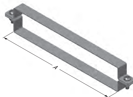
Обхватывающий зажим крышки канала СТЕ
