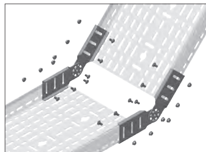
4 шт шарнирный соединитель для изменения уровня 4 шт болт М6х12 4 шт гайка М6.
