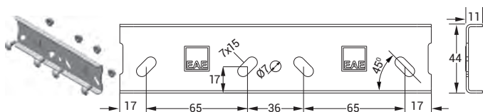
СОЕДИНИТЕЛЬНЫЙ ЭЛЕМЕНТ 040 СТЕ
