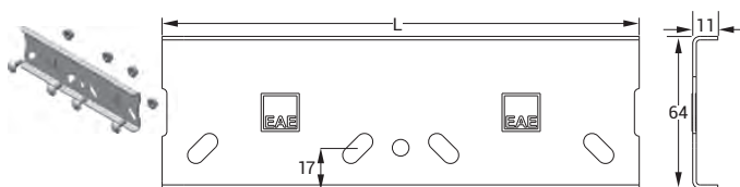
СОЕДИНИТЕЛЬНЫЙ ЭЛЕМЕНТ 060 СТЕ
