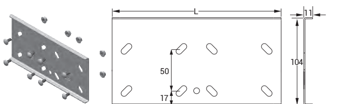
СОЕДИНИТЕЛЬНЫЙ ЭЛЕМЕНТ 100 СТЕ
