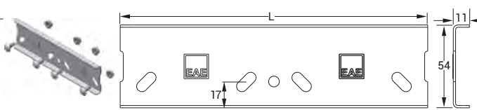
СОЕДИНИТЕЛЬНЫЙ ЭЛЕМЕНТ 050 СТЕ
